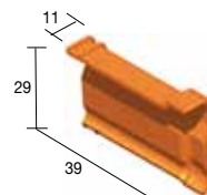
17 TAC Rechter gevelpan - 3 per lm - 3,08 kg
