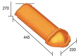
44 XT Eindnoordboom Résidence - 2,4 kg
