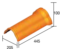
321 XT Ronde vorst Résidence + klem - 2,5 per lm - 3,6 kg
