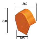
367 XT Begin-en eindvorst Résidence - 2,4 kg
