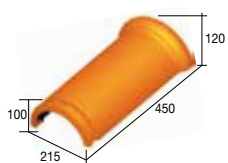
31 XT Ronde vorst - 2,5 per lm - 4,4 kg
