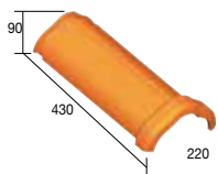
32 XT Noordboom Résidence - 3 per lm - 2,85 kg
