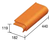
182 XT Shed-gevelpan - 2,5 per lm - 2,7 kg
